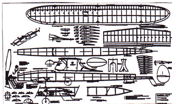
Lidgard, HI Ho, 1940
